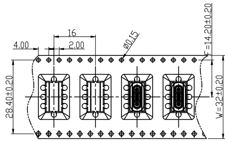
① 产品入载带示意图
