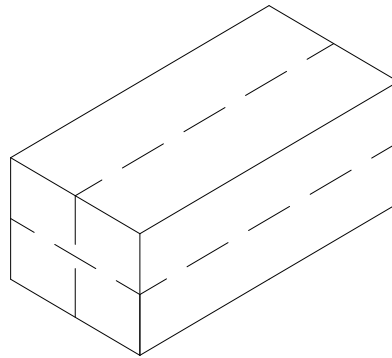
Export Carton: L580*W380*H240mm
