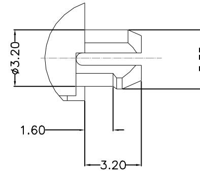
A(2:1)
