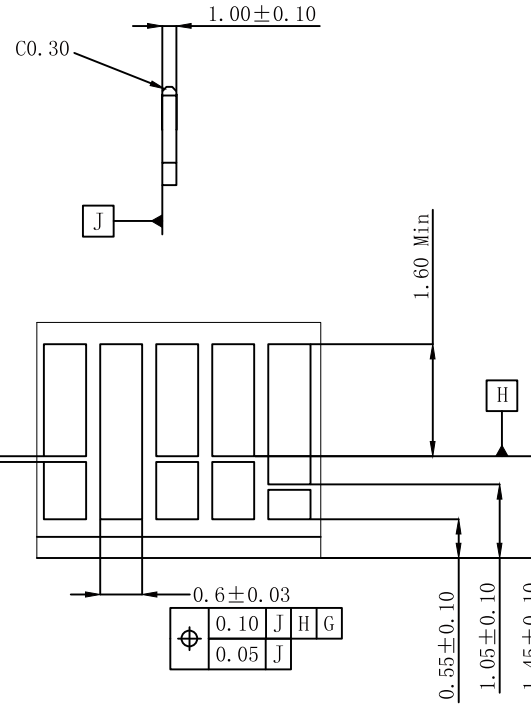
局部视图 D 比例 10 : 1
