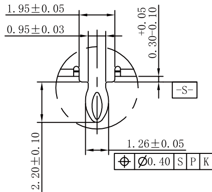
局部视图:A 比例 5:1
