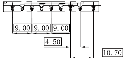
局部视图:B
